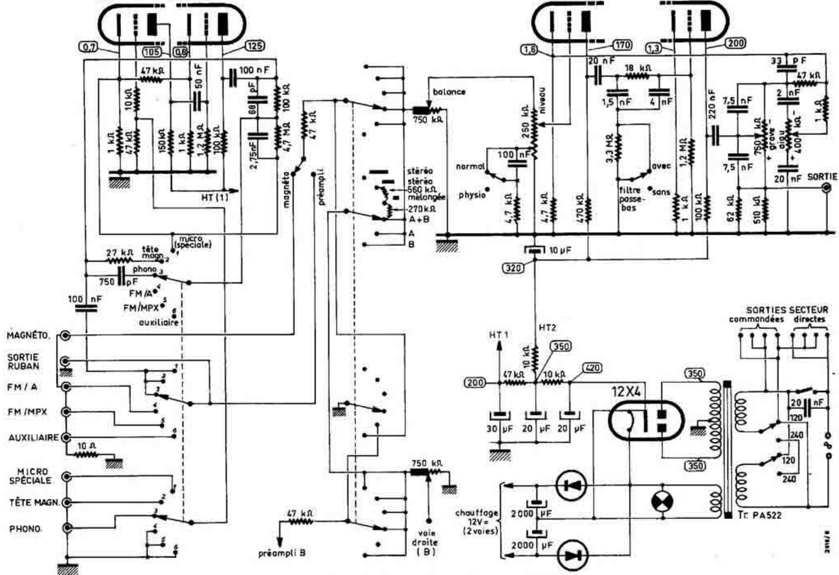
Schéma du préamplificateur PAS3.
