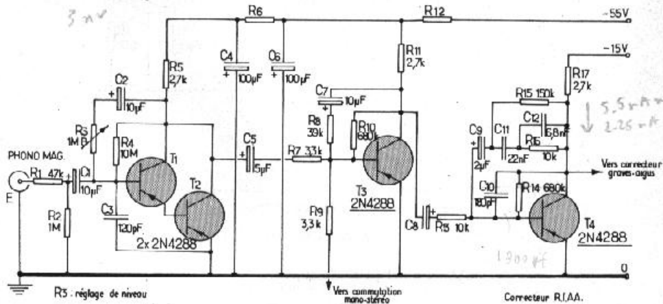
PARTIE DU PRÉAMPLIFICATEUR "CAMBRIDGE AUDIO" P.40
