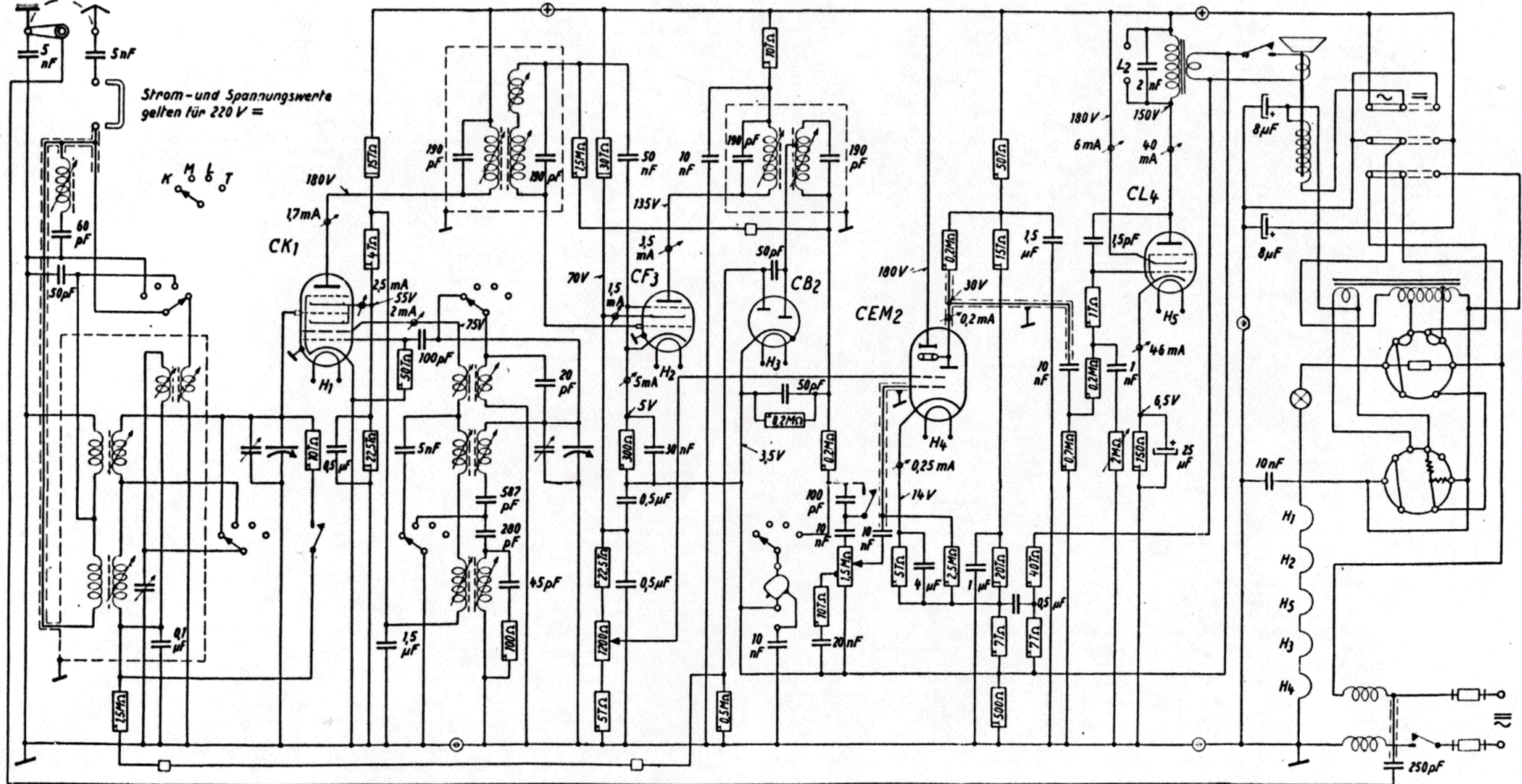
Siemens, Standard 75 GW, Allstrom, 1 Vorkreis, 4 Zwischenfrequenzkreise,
