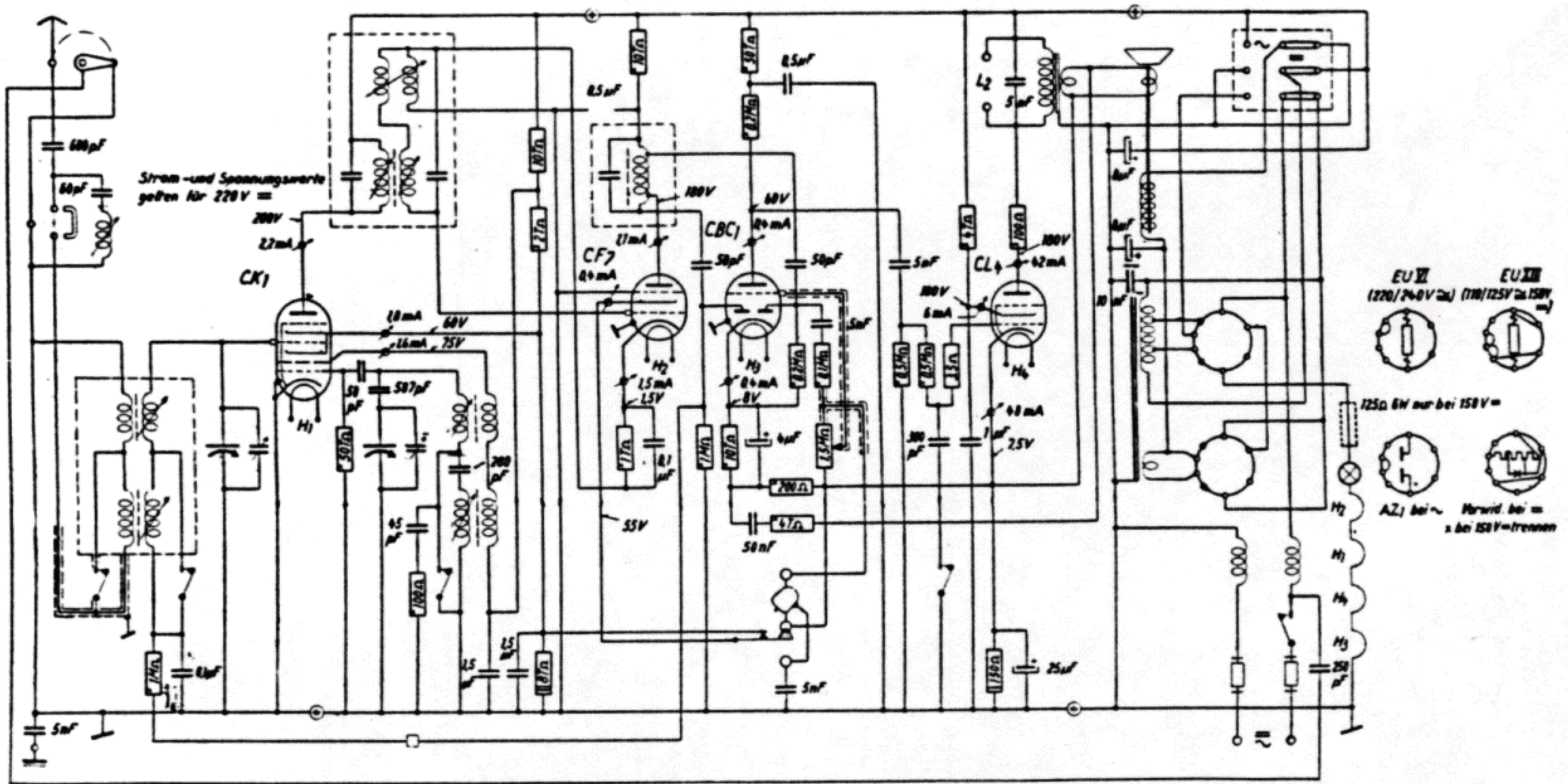
Siemens, Standard 74 GW, Allstrom, 1 Vorkreis
