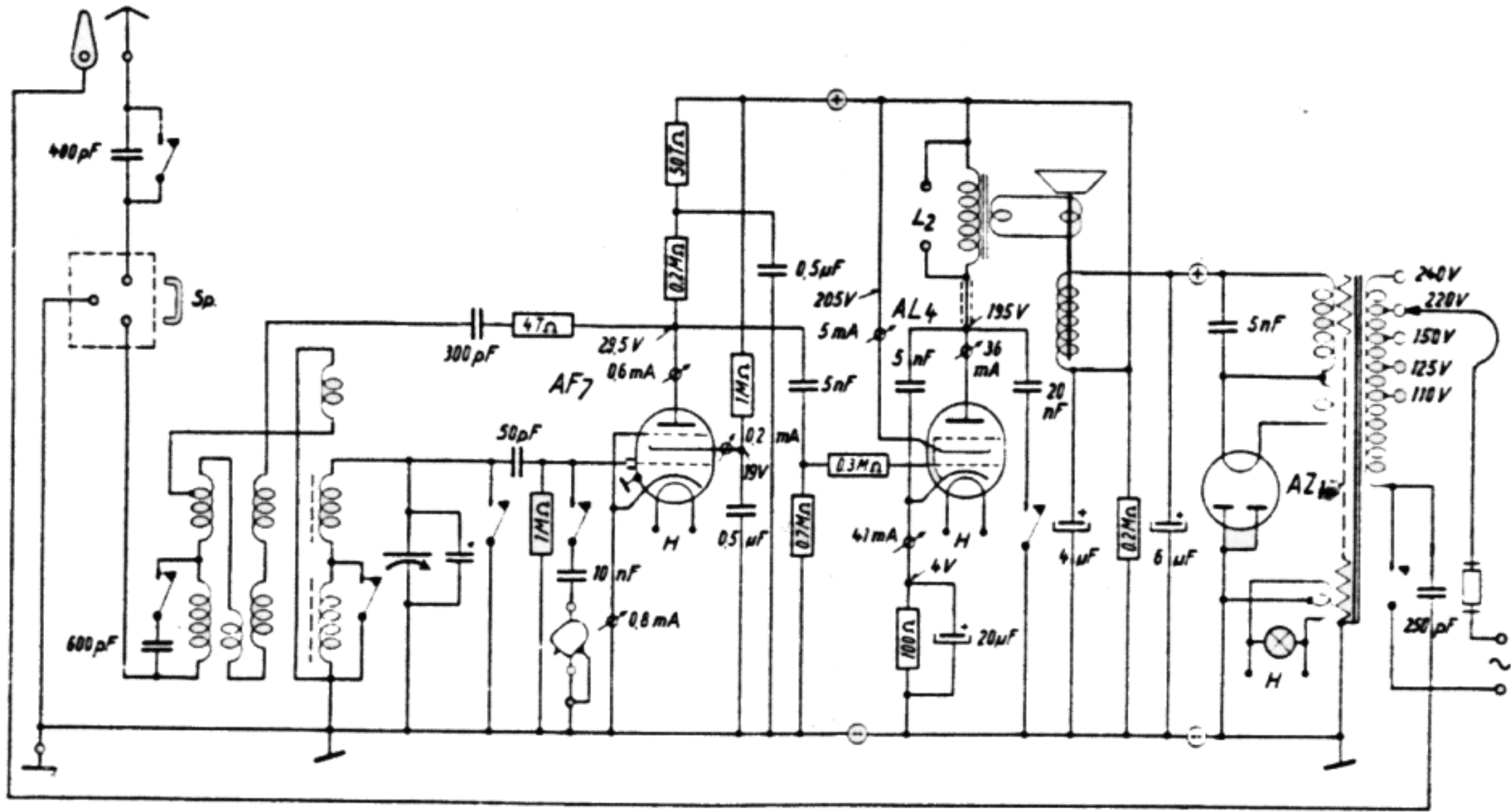
Siemens, Standard 72W, Wechselstrom, 1 Kreis,
