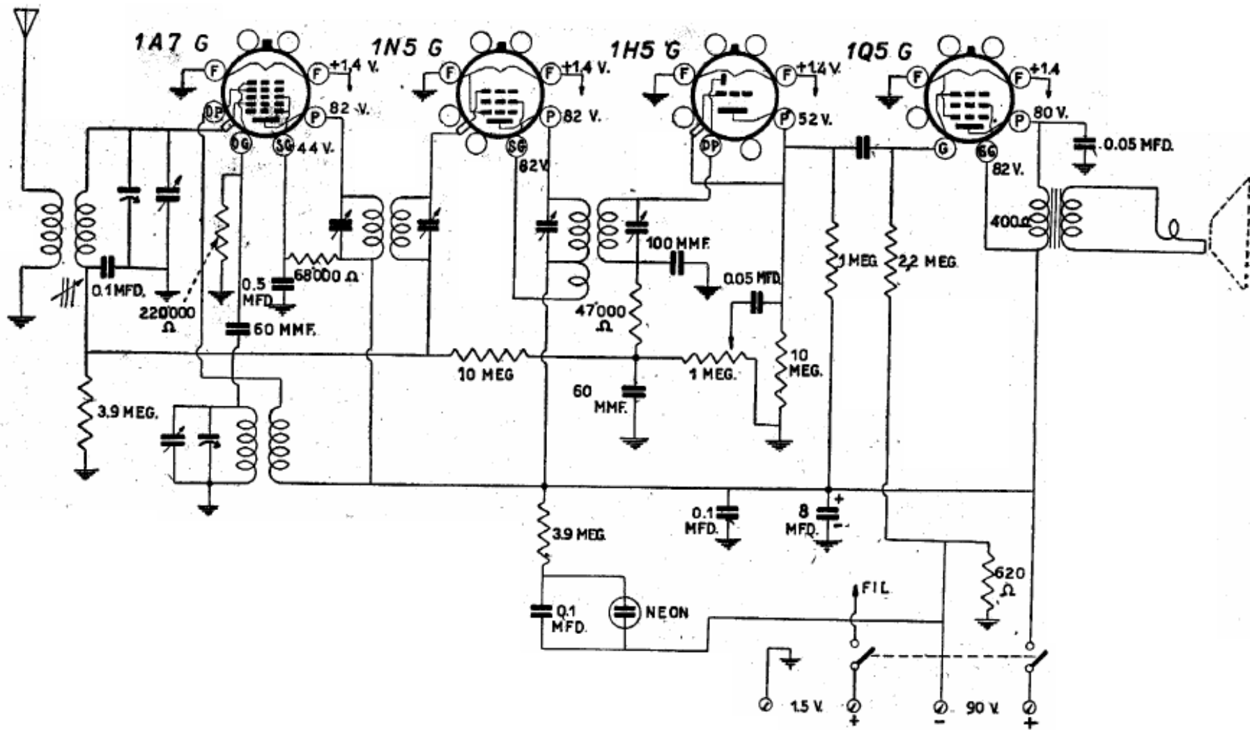
RCA mod. BT 42.
