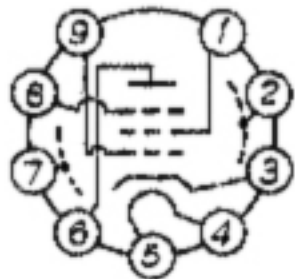
EF86
