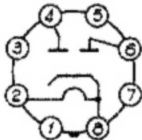
GZ34
